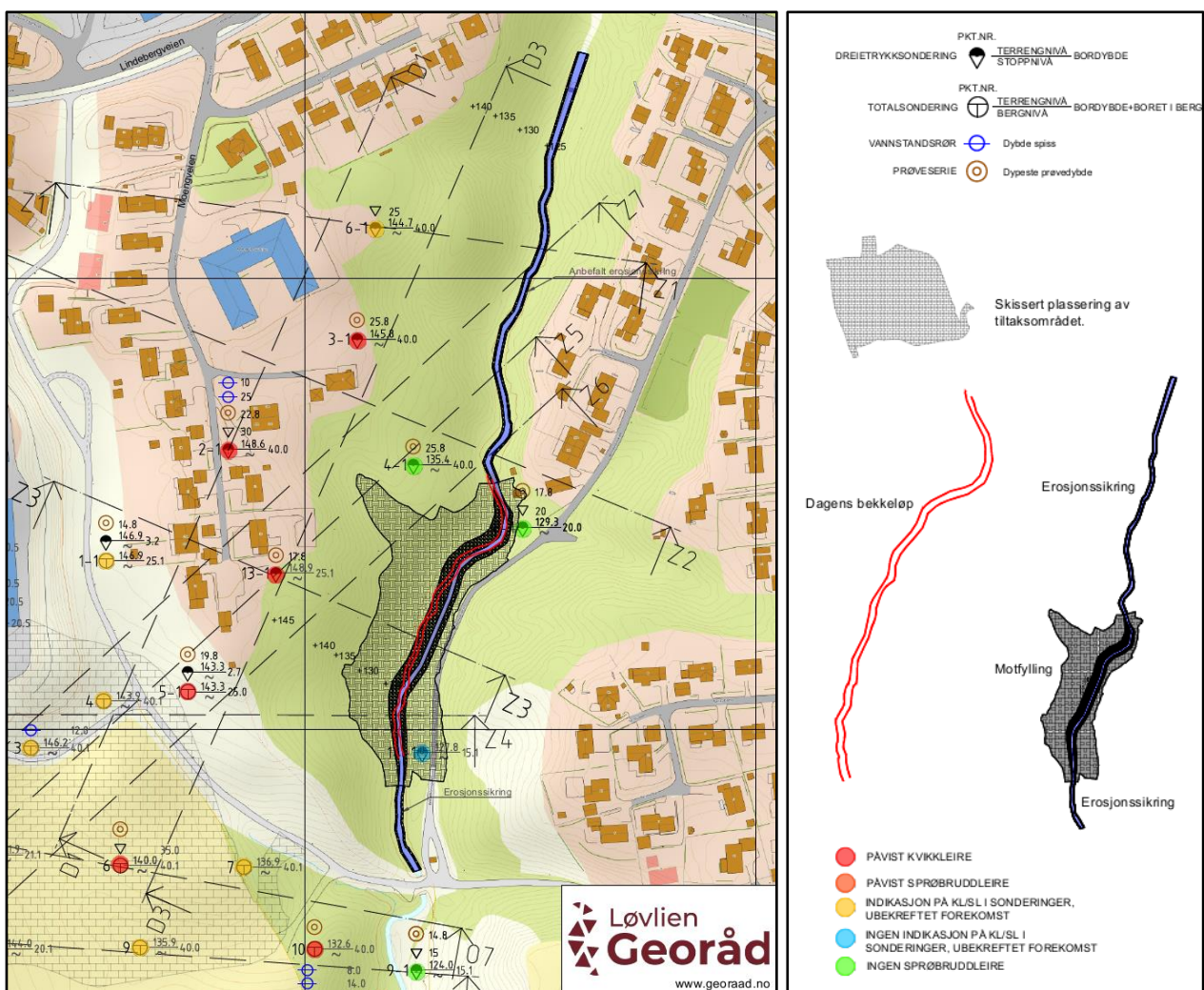
Skisse av fylling, erosjonssikring og omlegging av bekk. (Kilde: Løvlien Georåd, 20071 rapport nr. 2.)
