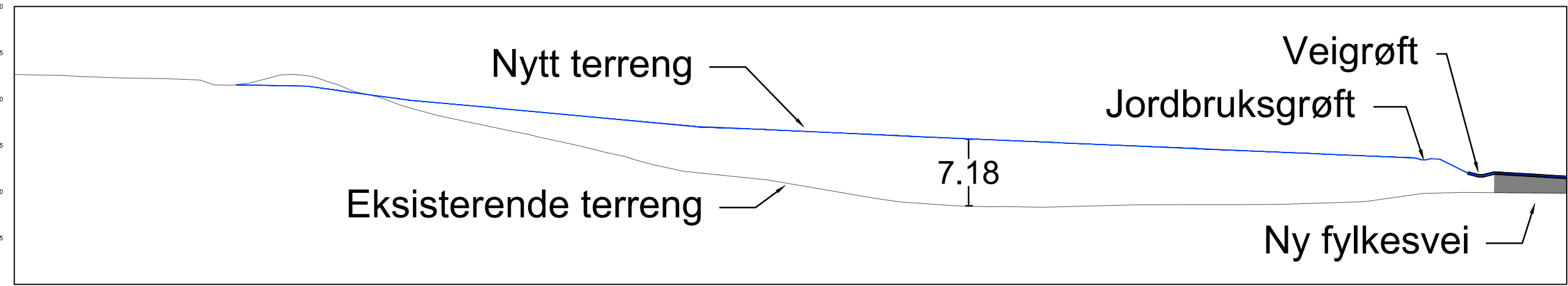
PROFIL: Profil 4
