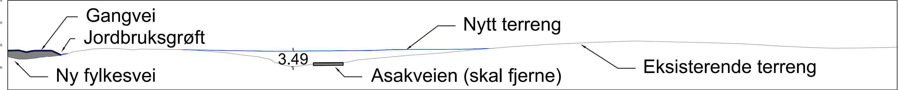
PROFIL: Profil 5
