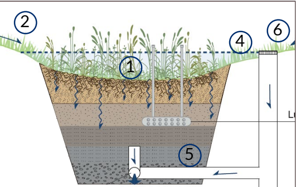
Figuren viser oppbygning av et regnbed/infiltrasjonsgrøft med viktige elementer markert. Illustrasjon: Oslo kommune/COWI.
